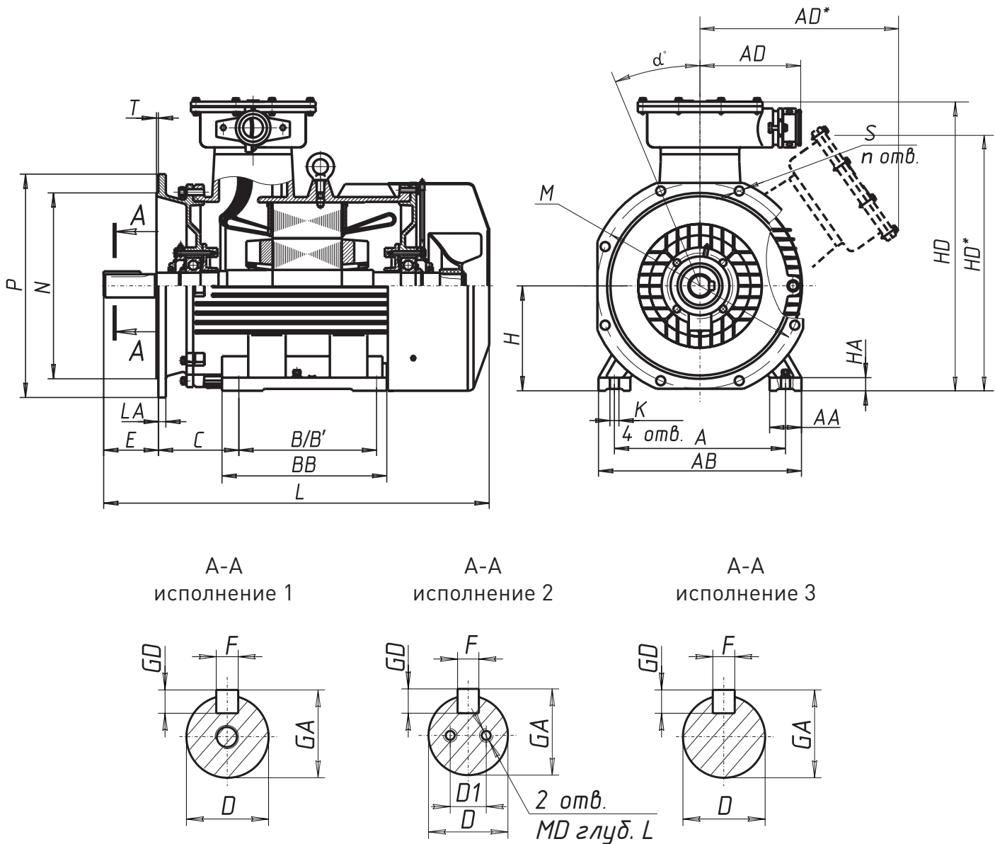
Монтажное исполнение IM 97..1
